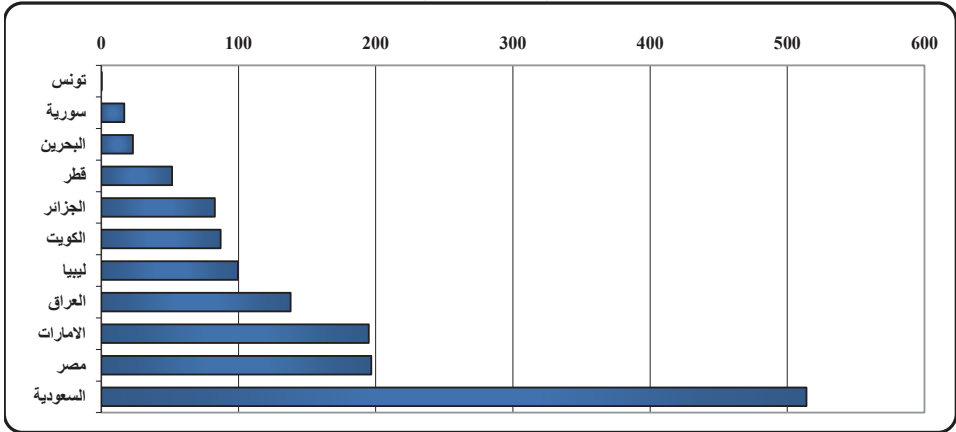
استهلاك الغازولين في الدول الأعضاء، 2020 - 2024 (ألف برميل / يوم)
