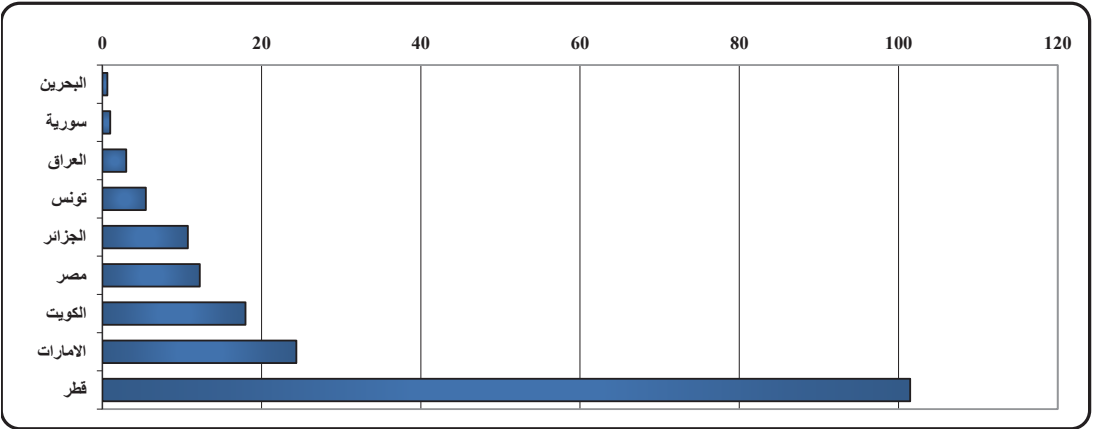
استهلاك وقود الطائرات في الدول الأعضاء، 2020 - 2024 (ألف برميل / يوم)
