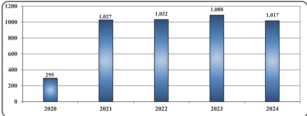
انتاج المشتقات النفطية الأخرى في الدول الأعضاء، 2024 - 2020 (ألف برميل / يوم)
