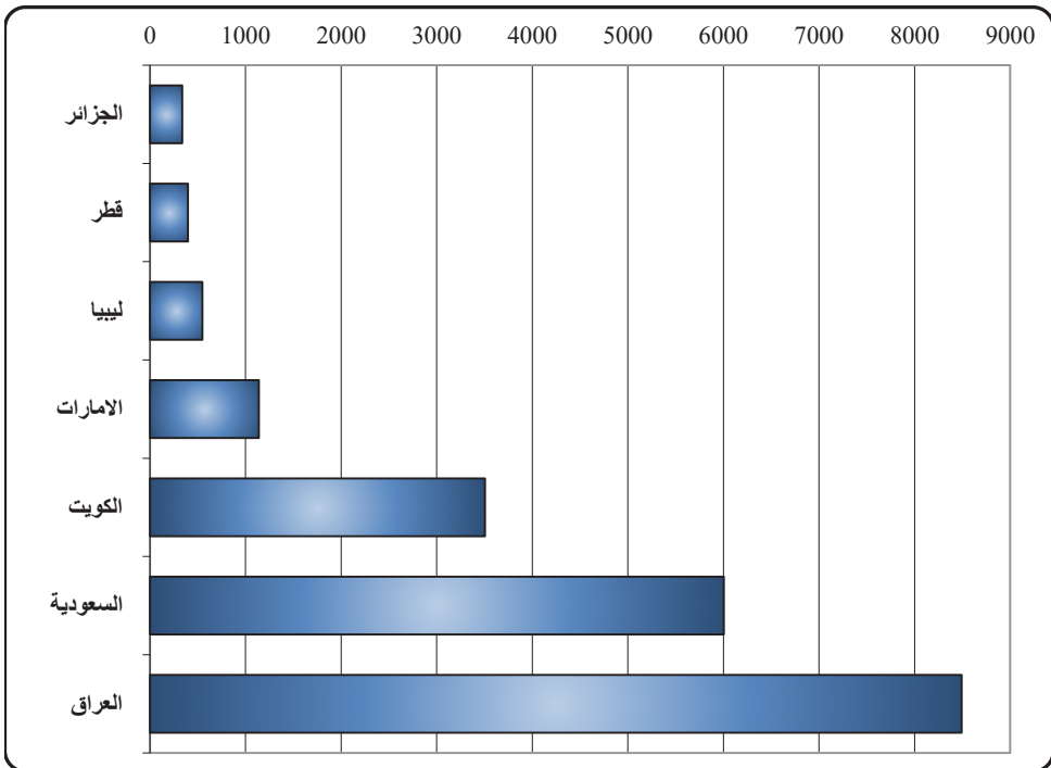
حمولة ناقلات النفط في الدول الأعضاء، عام 2024 (ألف طن ساكن)
