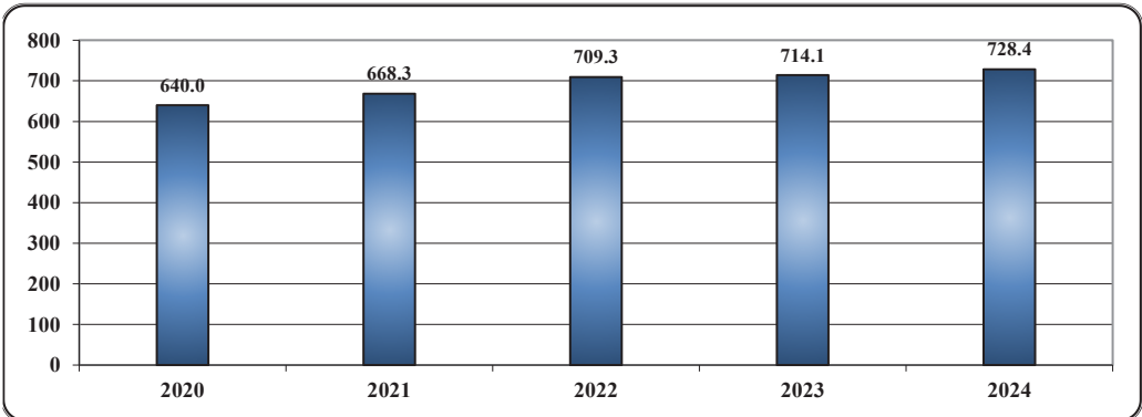
انتاج غاز البترول المسال في الدول الأعضاء، 2024 - 2020 (ألف برميل / يوم)
