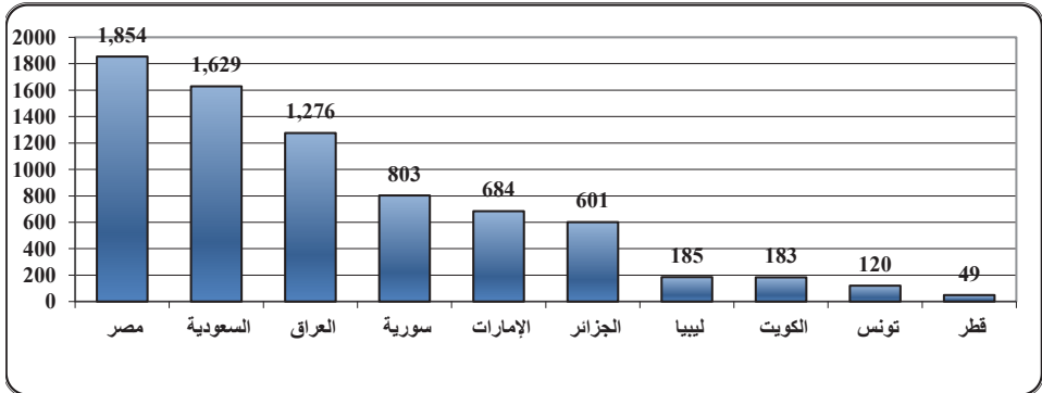
طول خطوط شبكة انابيب المشتقات النفطية (في نهاية عام 2024) (ميل)
